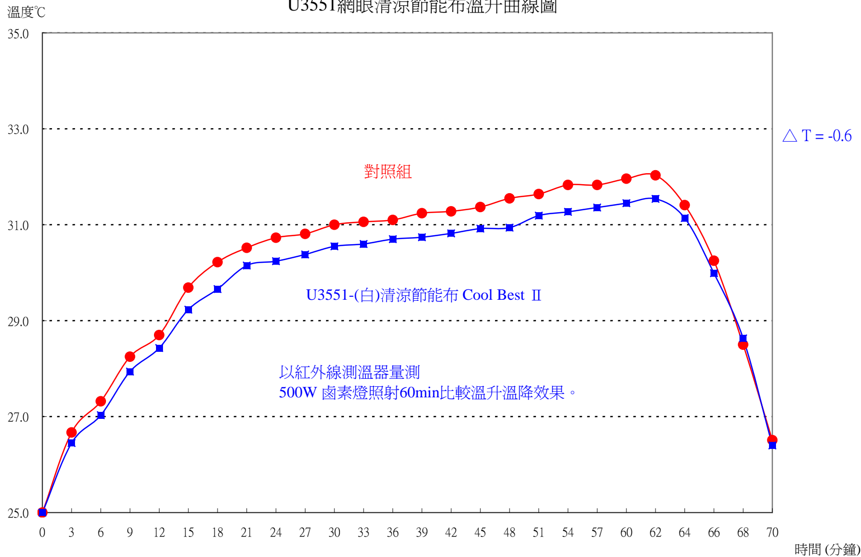
U3551網眼清涼節能布溫升曲線圖
